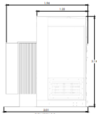
ELEVATION B-B
