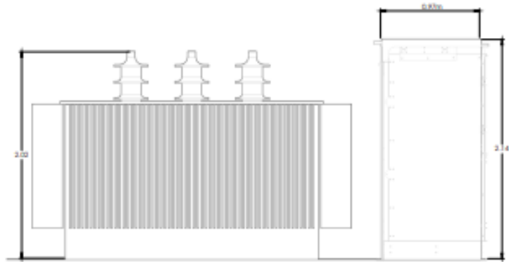
ELEVATION A-A
